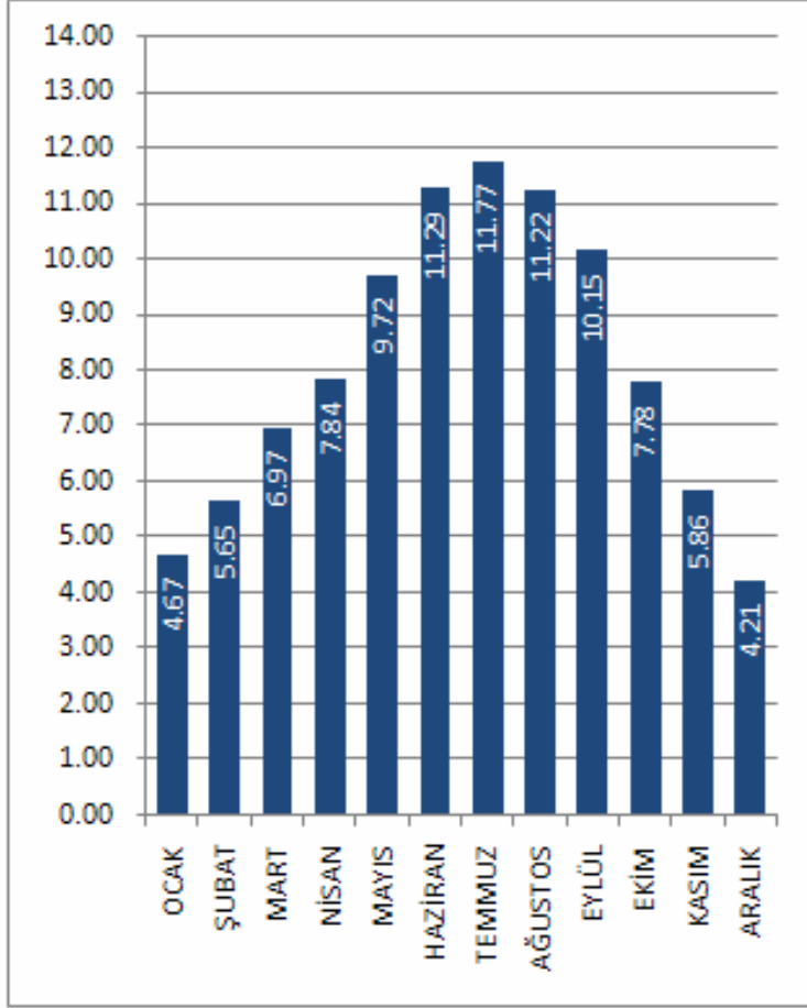
ADANA İLİ GÜNEŞLENME SÜRESİ DEĞERLERİ (Saat)
