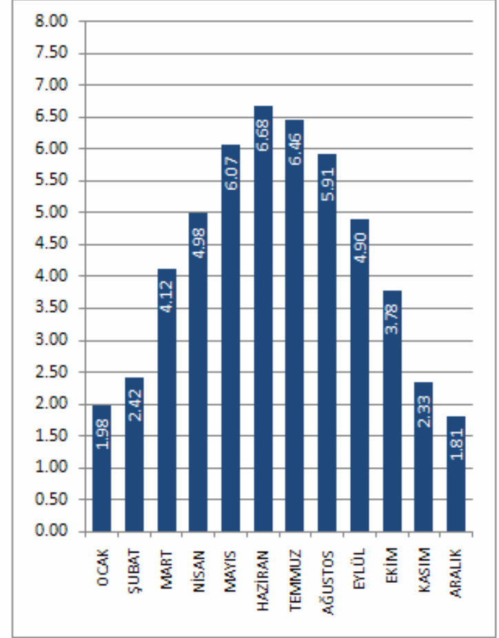
ADANA İLİ GLOBAL RADYASYON DEĞERLERİ (KWh/m 2 -gün)
