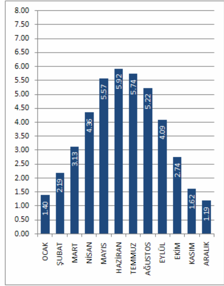
İSTANBUL İLİ GLOBAL RADYASYON DEĞERLERİ (KWh/m 2 -gün)
