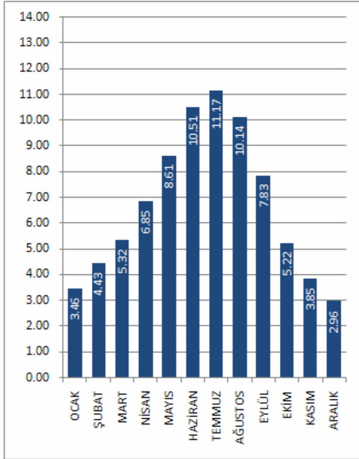
İSTANBUL İLİ GÜNEŞLENME SÜRESİ DEĞERLERİ (Saat)
